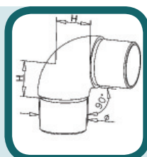
Угловой элемент 90° Ø38, Ø50
