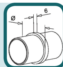
Соединительный элемент Ø38, Ø50
